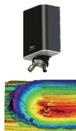
干渉式顕微鏡による表面性状測定
